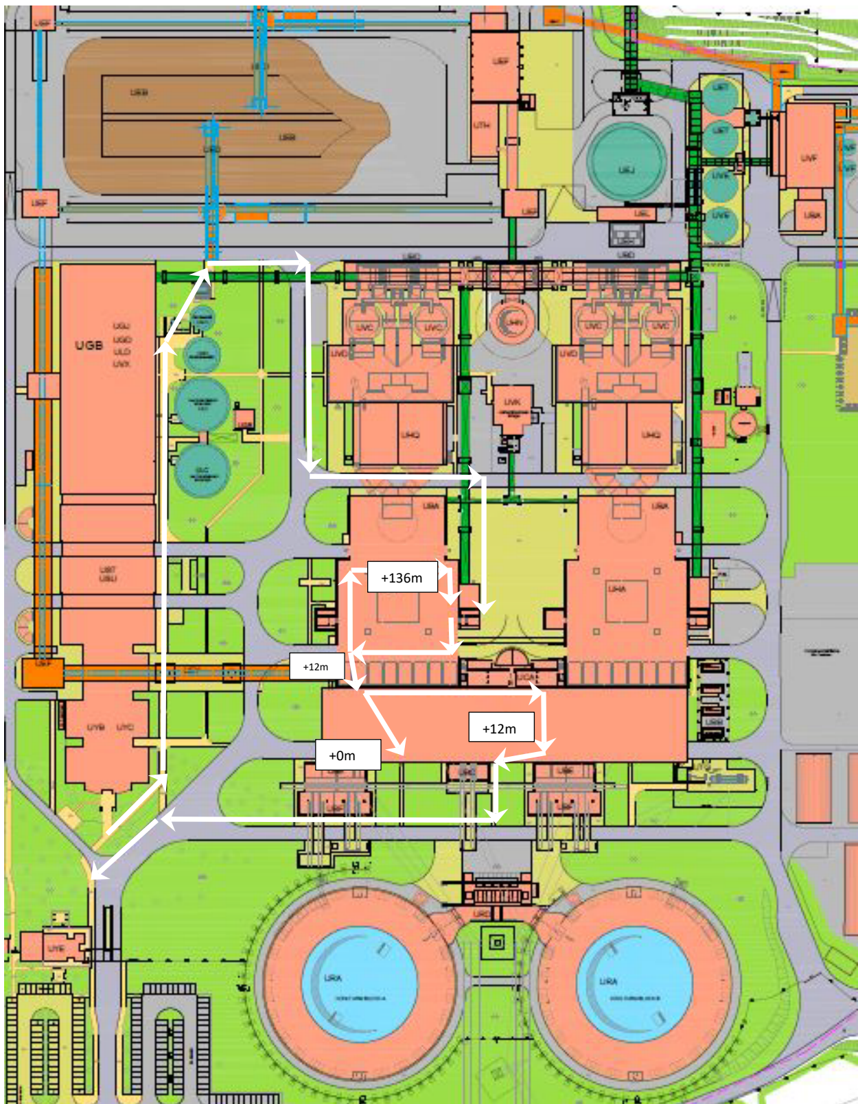
Anlage 2: Routenverlauf Besucherweg
